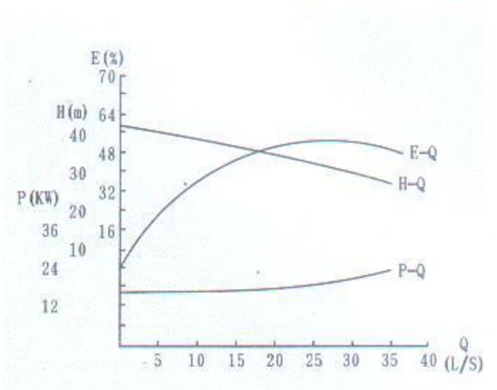
ZW100-100-30
