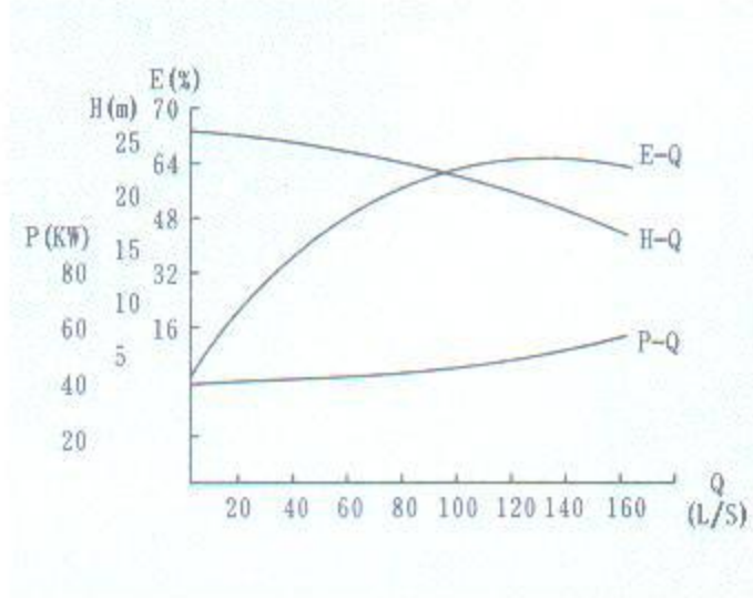
ZW250-420-20
