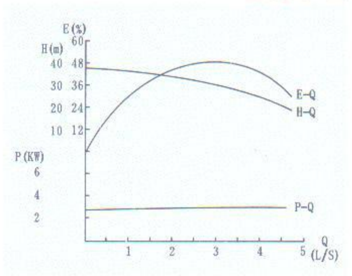
ZW32-9-30
