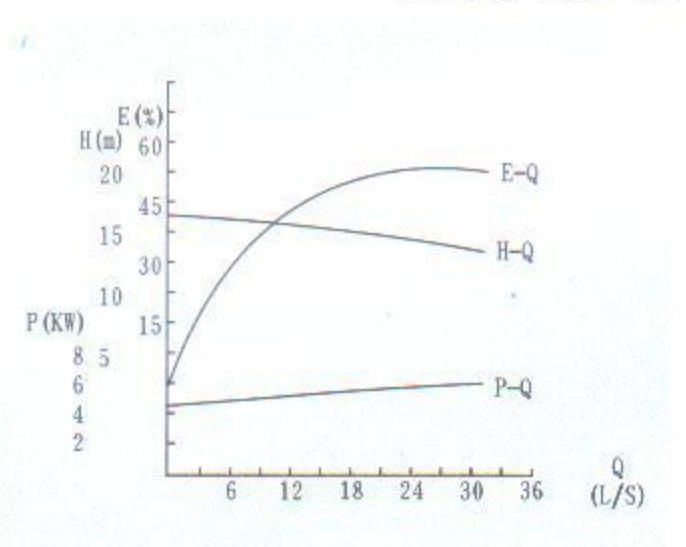
ZW100-100-15
