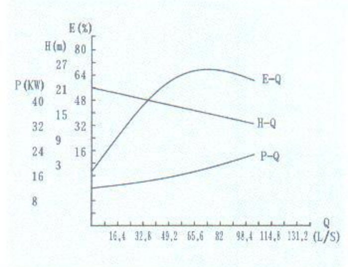
ZW200-280-14
