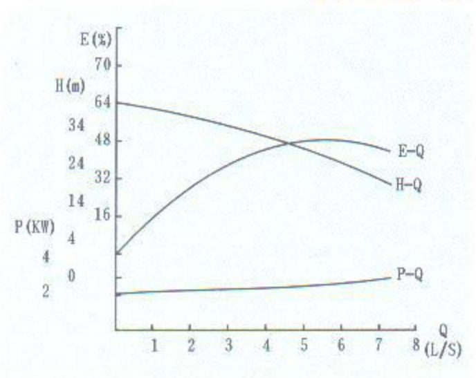
ZW40-15-30 ZW50-15-30
