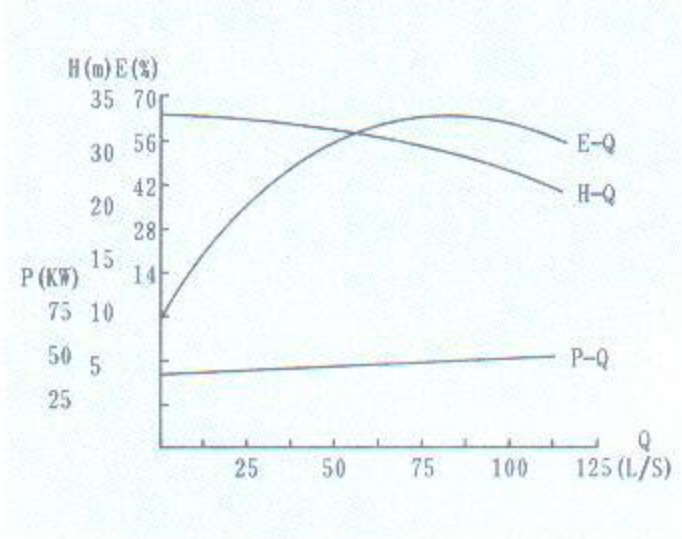
ZW200-280-28
