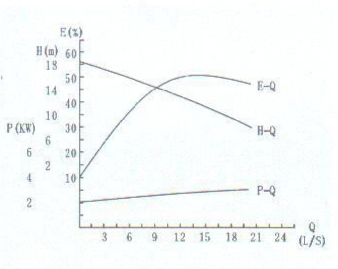
ZW65-30-18 ZW80-40-16
