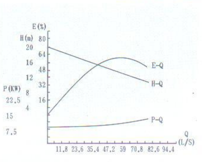
ZW150-180-30
