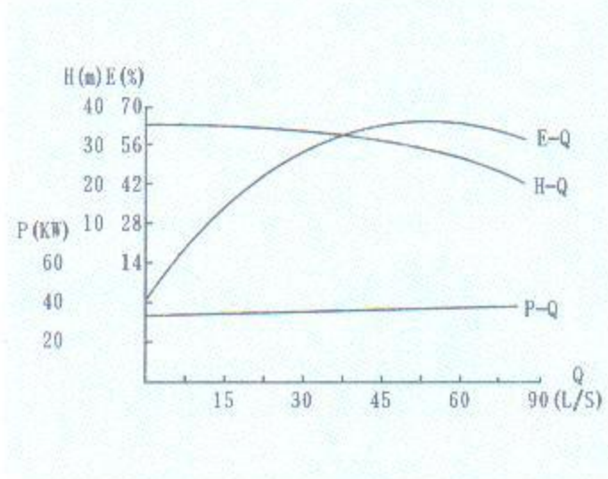
ZW150-180-30
