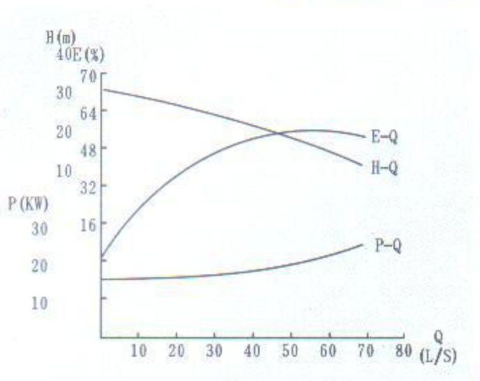
ZW150-180-20
