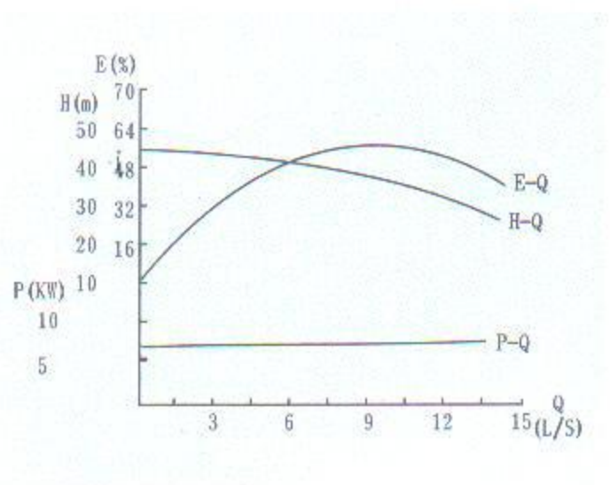
ZW65-25-40
