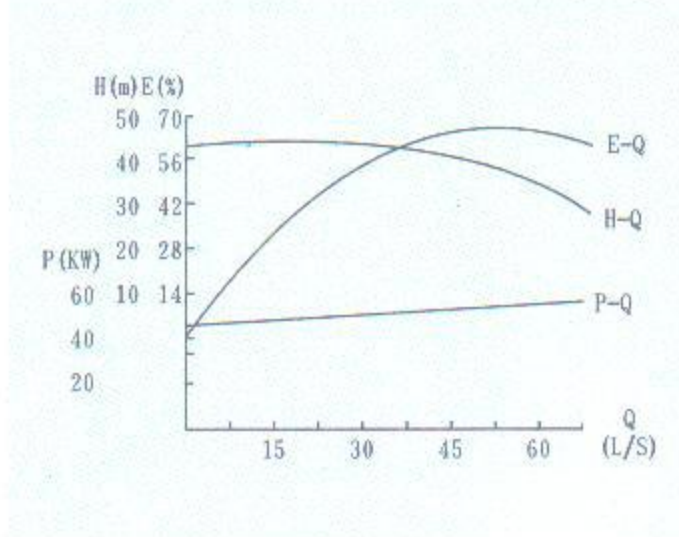
ZW150-180-38
