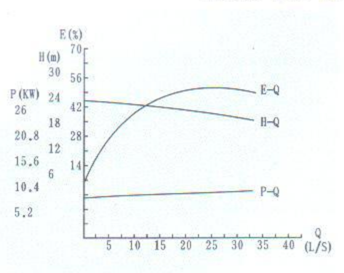
ZW100-100-20
